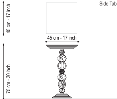
Dimensioni / Dimensions L. 45 x P. 45 x H. 75 cm - L. 17 x W. 17 x H. 30 inch
